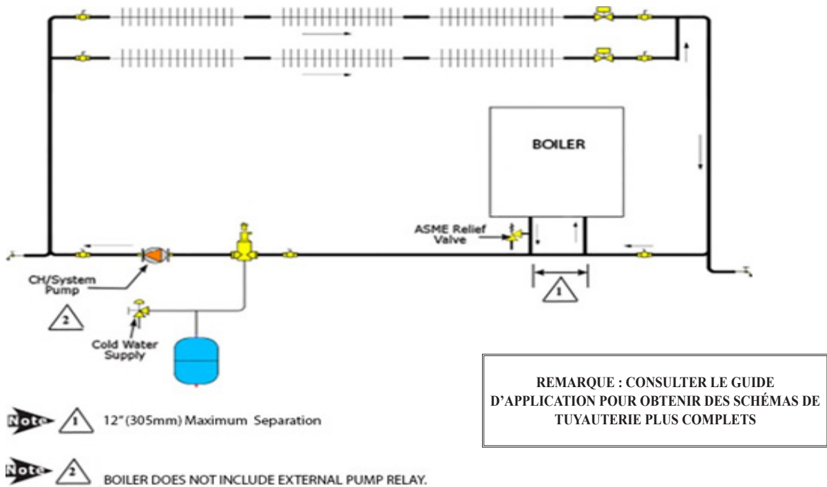
FIGURE 6-6 Configuration de base de la tuyauterie du système
