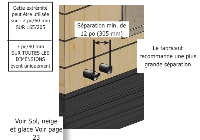
FIGURE 5-25 – Tuyau double horizontal, évacuation et prise d’air
