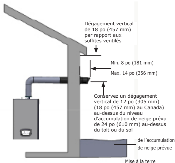
FIGURE 5-6 – Évén coaxial pour mur latéral PEUT ÊTRE UTILISÉ SUR TOUTES LES TAILLES
