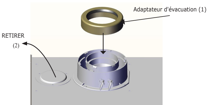
Figure 5-16 – Adaptateur coaxial à tuyau double pour les modèles de chaudières 205
