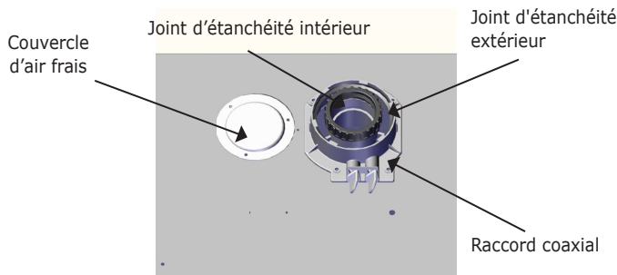
Figure 5-15 – Adaptateur coaxial à tuyau double pour les modèles de chaudières 205
