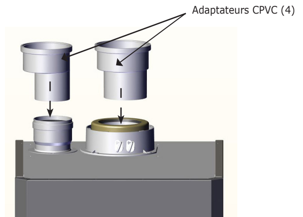
Figure 5-18 – Adaptateur de tuyau double en CPVC pour les modèles de chaudières 205
