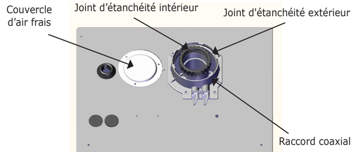
Figure 5-11 – Adaptateur de tuyau double pour les modèles de chaudières 150
