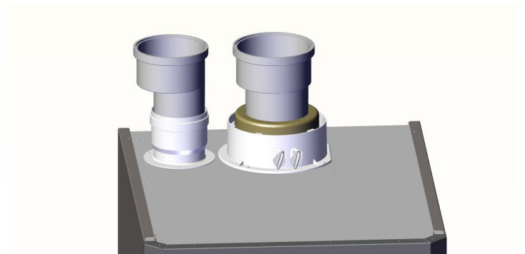
Figure 5-19 – Adaptateur de tuyau double en CPVC pour les modèles de chaudières 205
