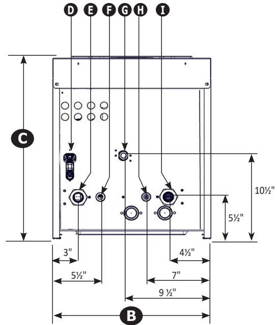
205 COMBI Vue de dessous Dimensions
