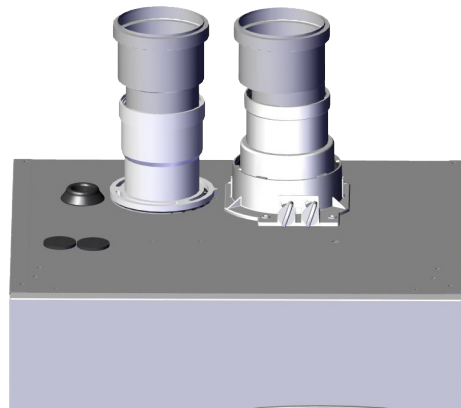
Figure 5-14 – Adaptateur de tuyau double en CPVC pour les modèles de chaudières 150
