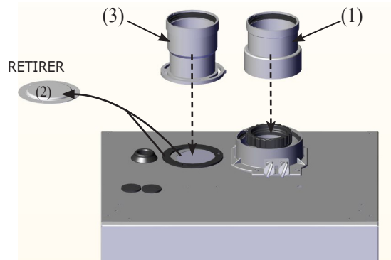
Figure 5-13 – Adaptateur de tuyau double en polypropylène pour les modèles de chaudières 150
