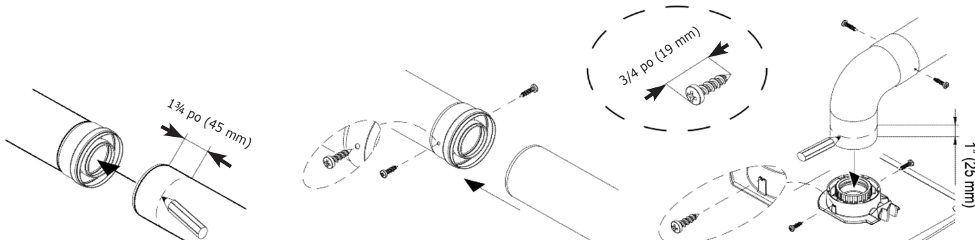
FIGURE 5-4 – Évén coaxial pour installation sur le toit PEUT ÊTRE UTILISÉ SUR TOUTES LES TAILLES
